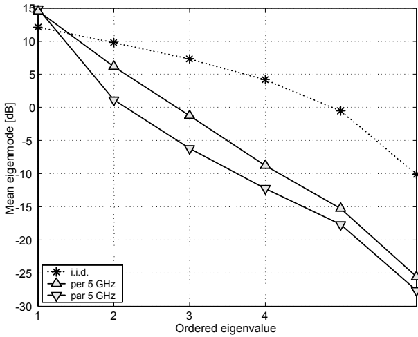
Fig. 3. Ordered eigenvalues.
